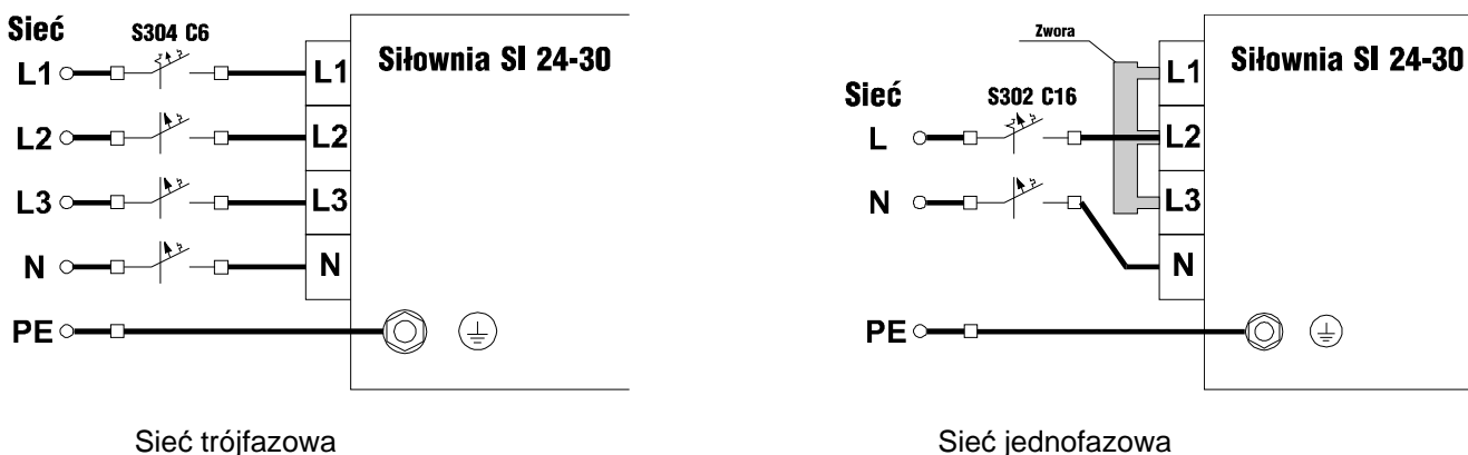
Rys.5 Schemat podłączenia zasilania siłowni SI24-30.
