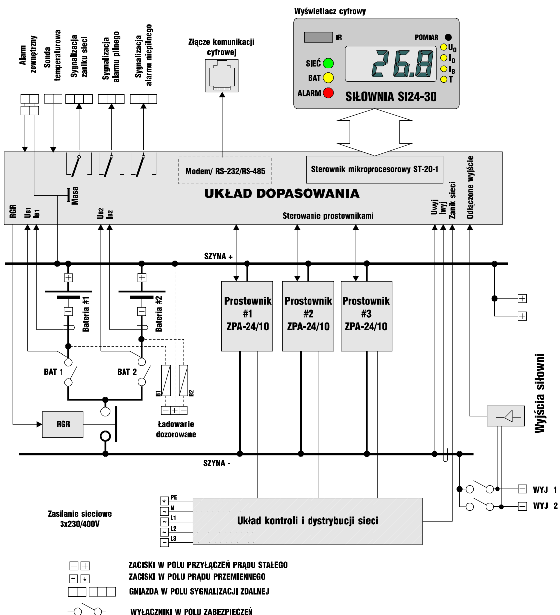
Rys. 3. Schemat blokowy siłowni SI24-30-31
