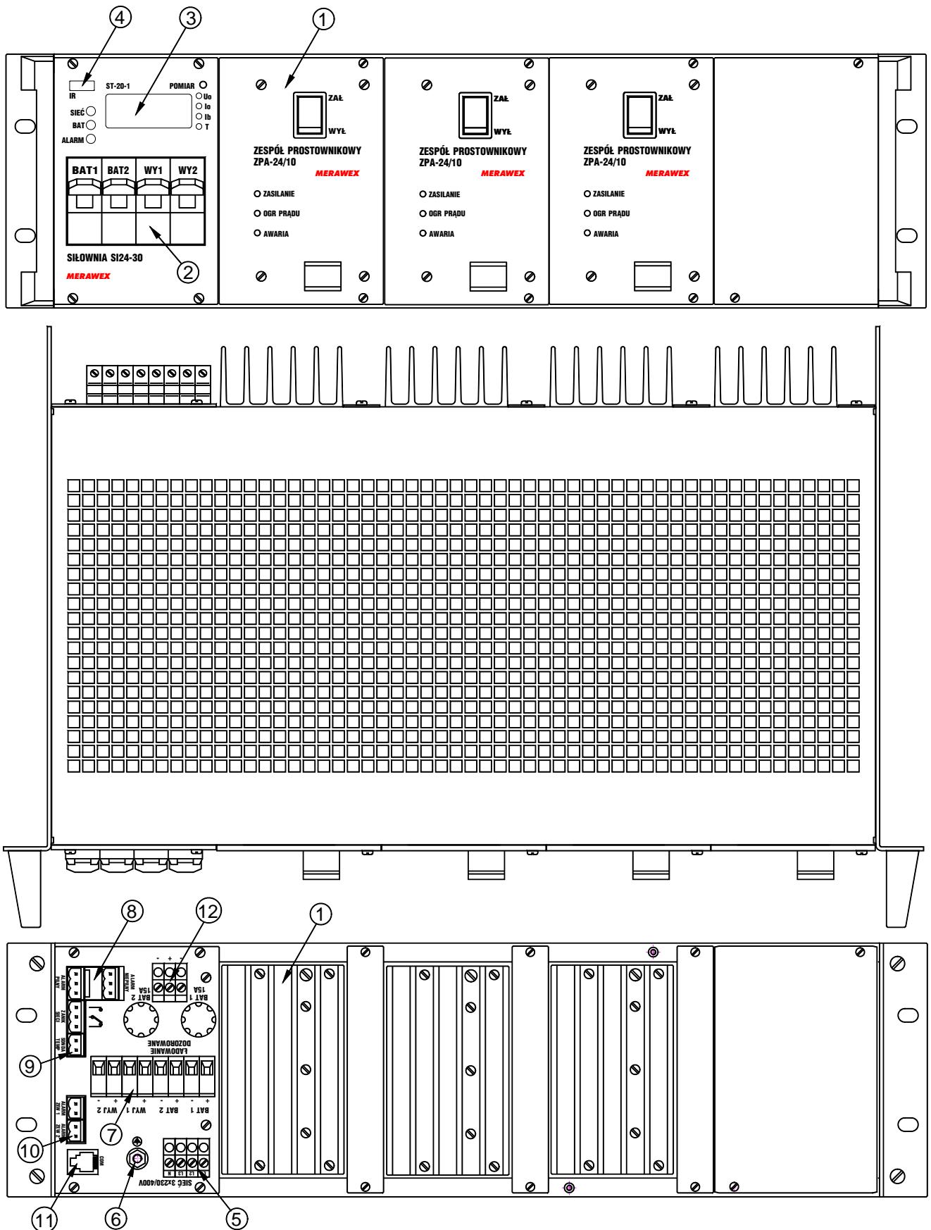
Rys.2. Wygląd zewnętrzny siłowni SI24-30-31 (urządzenie w pełnej konfiguracji – zawiera opcjonalne wejście zewnętrznego obwodu ładowania dozorowanego).
