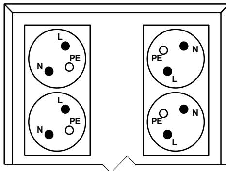
Rysunek 10: Układ wyprowadzeń gniazd wyjściowych SINLINE w wersji Tower
